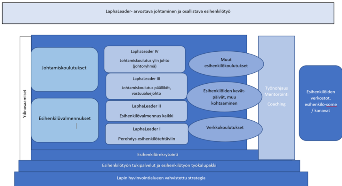
Kuva 5. Lapha Leader-malli.
